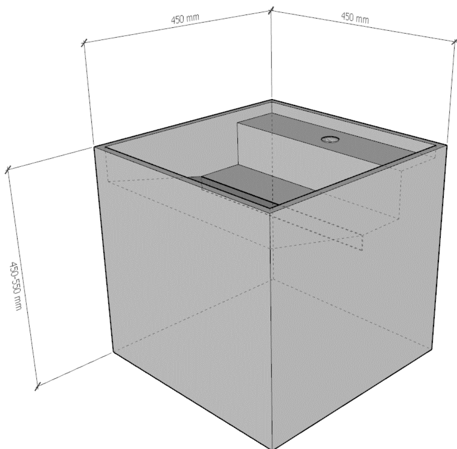
Раковина «Cube» підвісна з полицею
