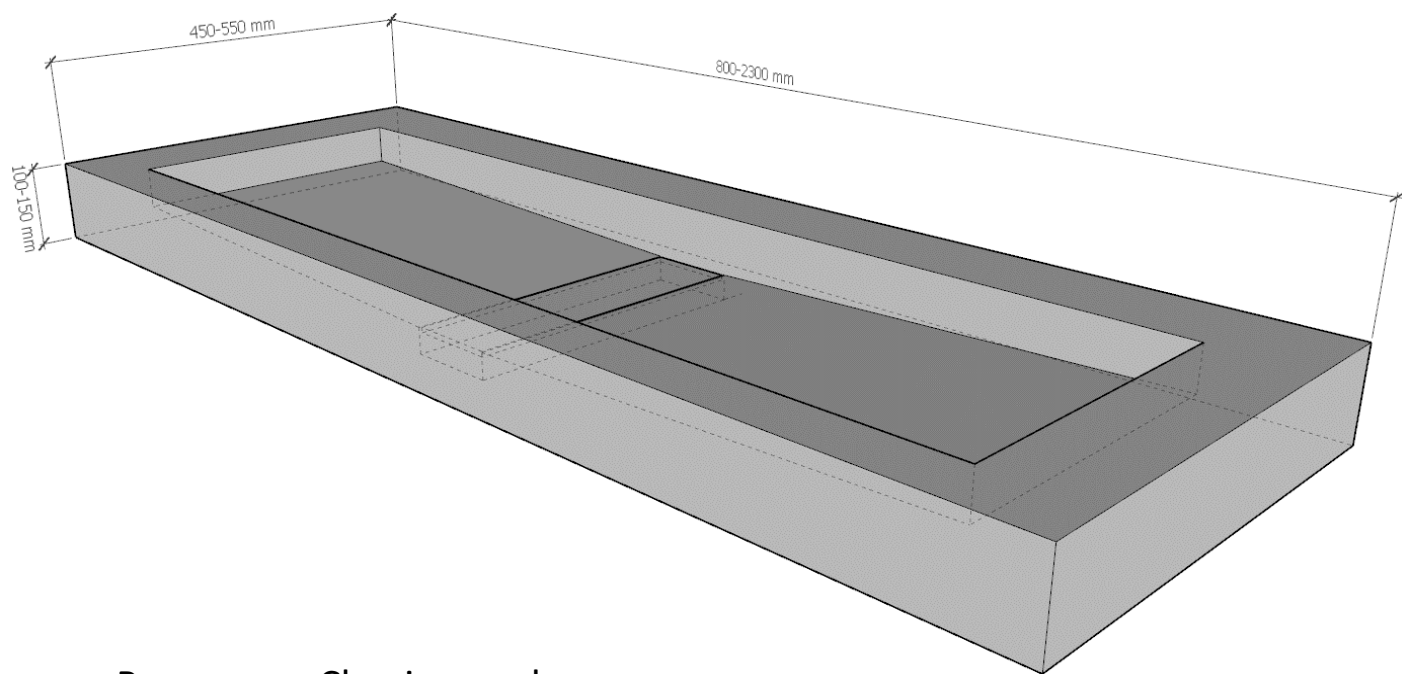
Раковина «Classic grand»
