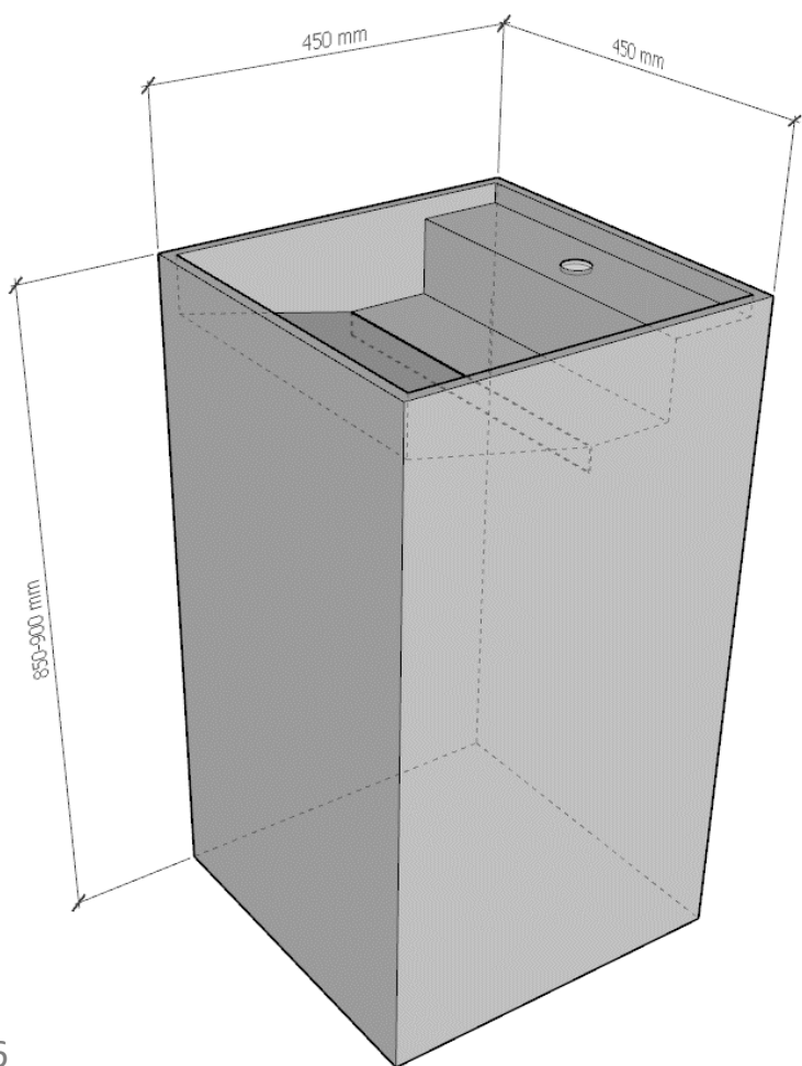
Раковина «Cube» з полицею
